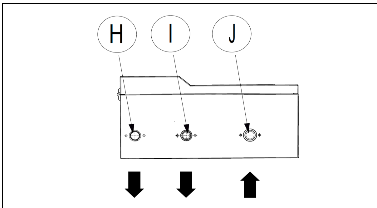
Rys. 10: Przyłącza hydrauliczne jednostki wewnętrznej pompy ciepła EUROS ATMO.
