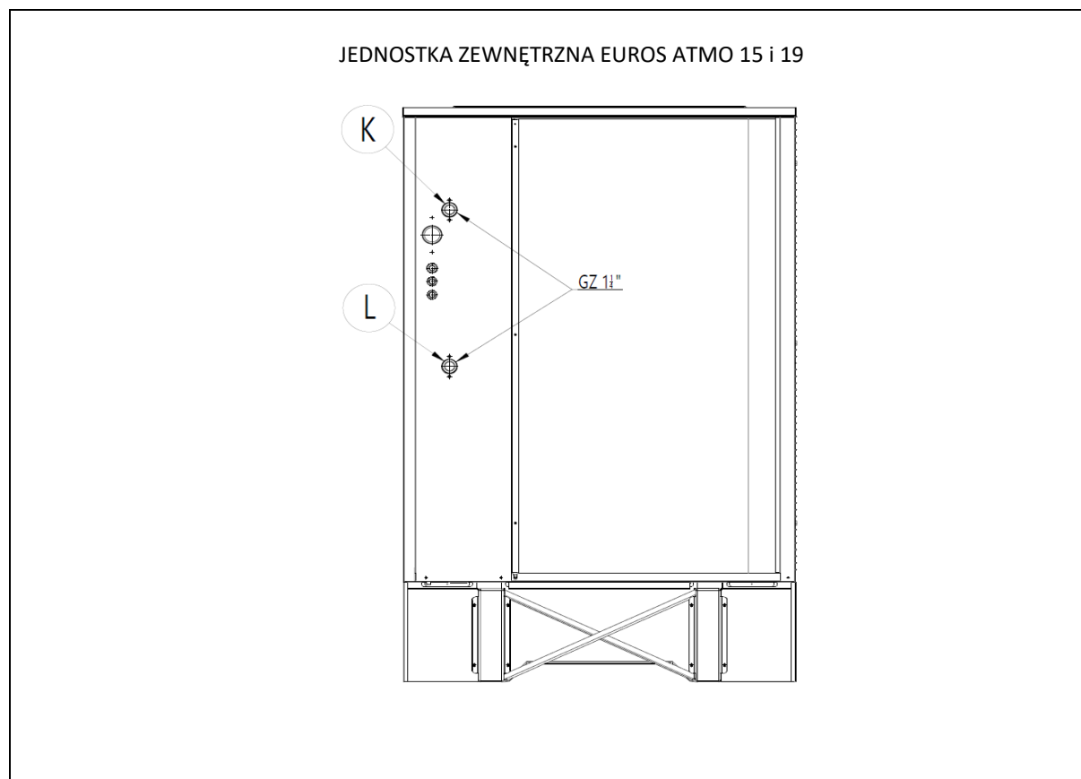
Rys. 11: Przyłącza hydrauliczne jednostki zewnętrznej pompy ciepła EUROS ATMO 15 i 19.
