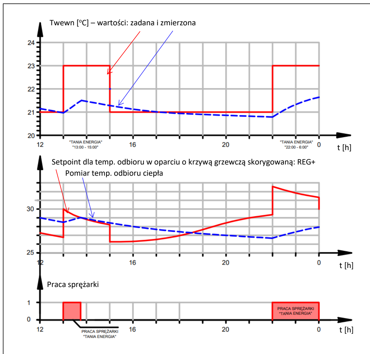
Rys. 18: Automatyczna zmiana temperatury zadanej w trybie ECO z wykorzystaniem mechanizmu REG+.
