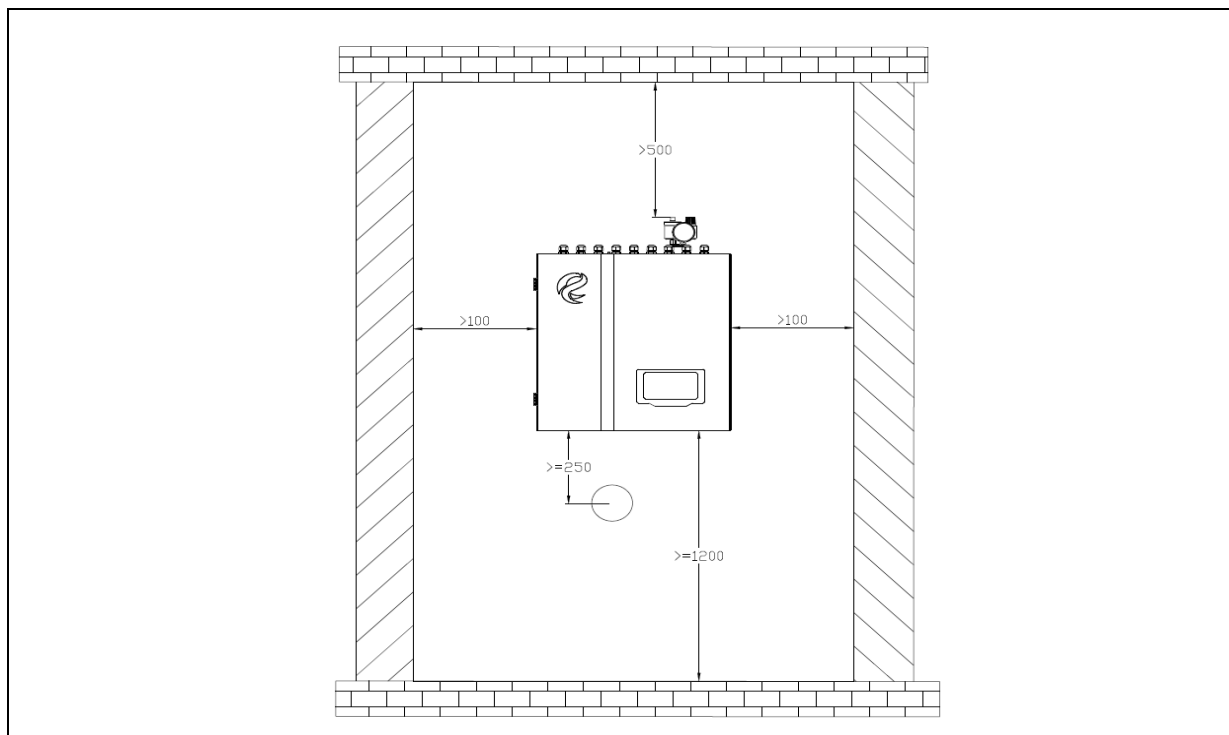
Rys. 8: Ograniczenia dotyczące miejsca ustawienia jednostki wewnętrznej pompy ciepła EUROS ATMO (wymiar w mm).
