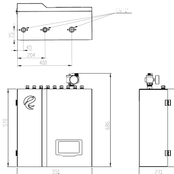
Rys. 5: Gabaryty jednostki wewnętrznej pompy ciepła EUROS ATMO.
