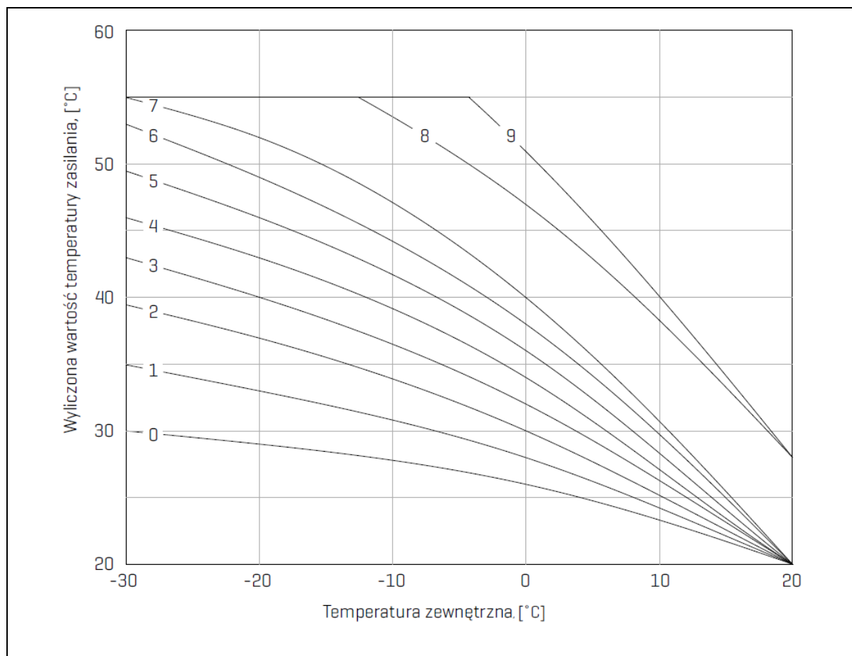
Rys. 14: Wykres krzywych grzewczych.
