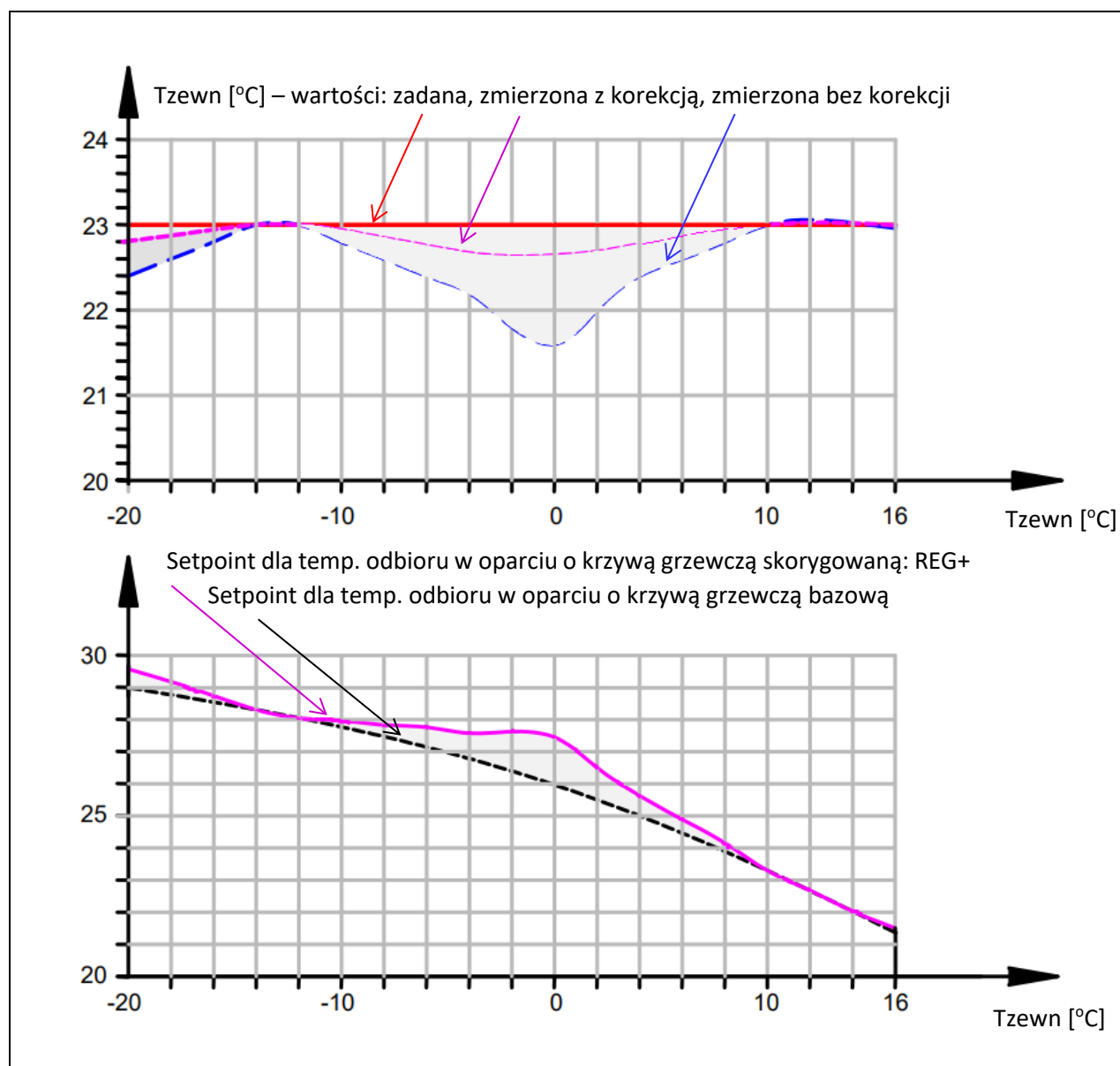
Rys. 16: Oddziaływanie mechanizmu REG+ na krzywą grzewczą.
