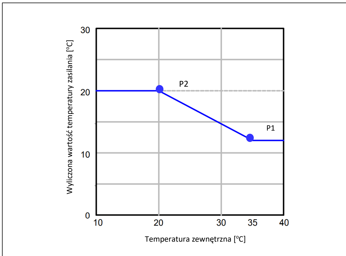
Rys. 15: Wykres krzywej chłodzenia.
