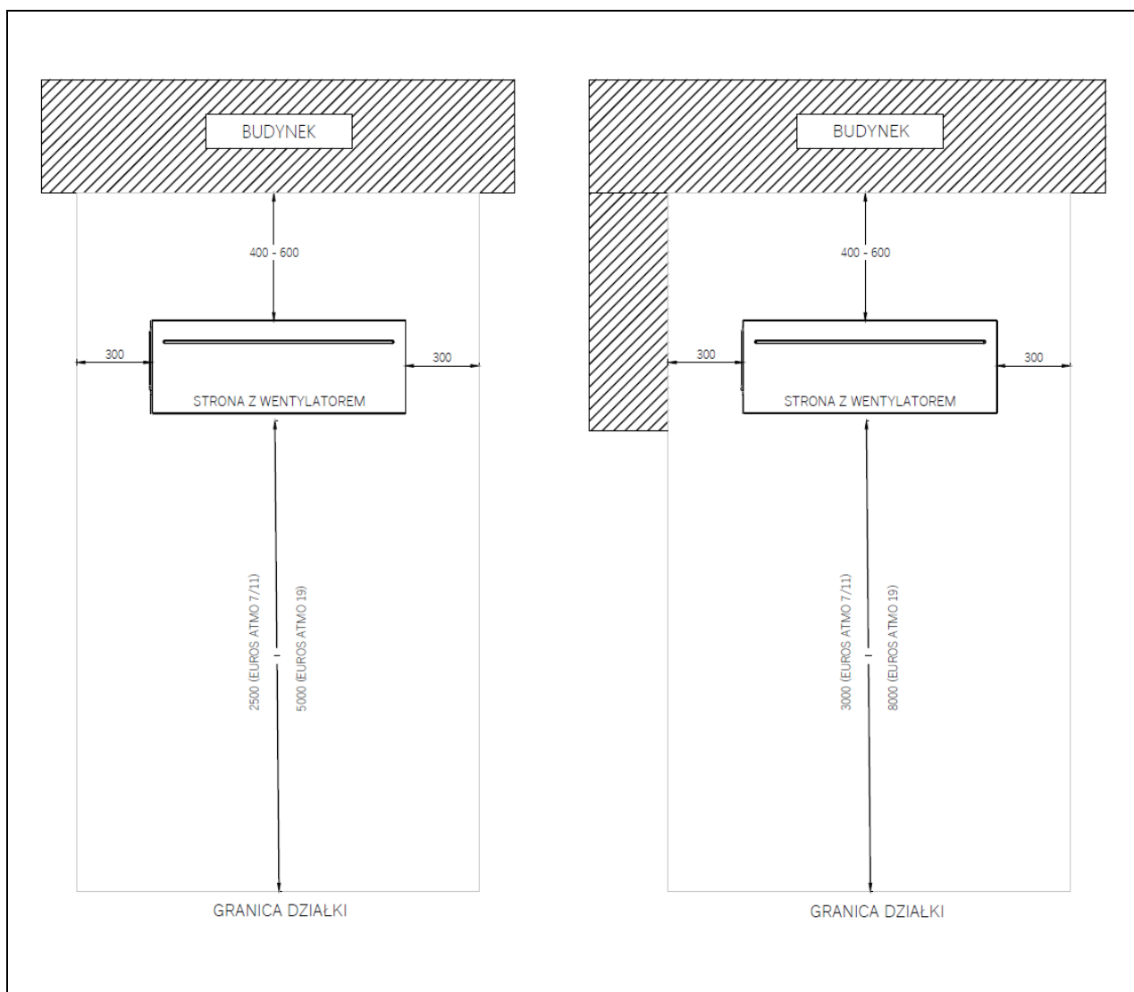
Rys. 9: Ograniczenia dotyczące miejsca ustawienia jednostki zewnętrznej pompy ciepła EUROS ATMO (wymiały w mm).
