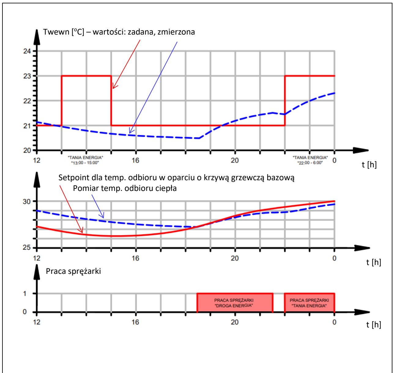
Rys. 17: Automatyczna zmiana temperatury zadanej w trybie ECO bez wykorzystania mechanizmu REG+.
