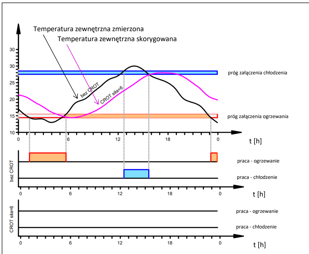
Rys. 19: Kontrola progu załączenia ogrzewania i chłodzenia – mechanizm CROT.
