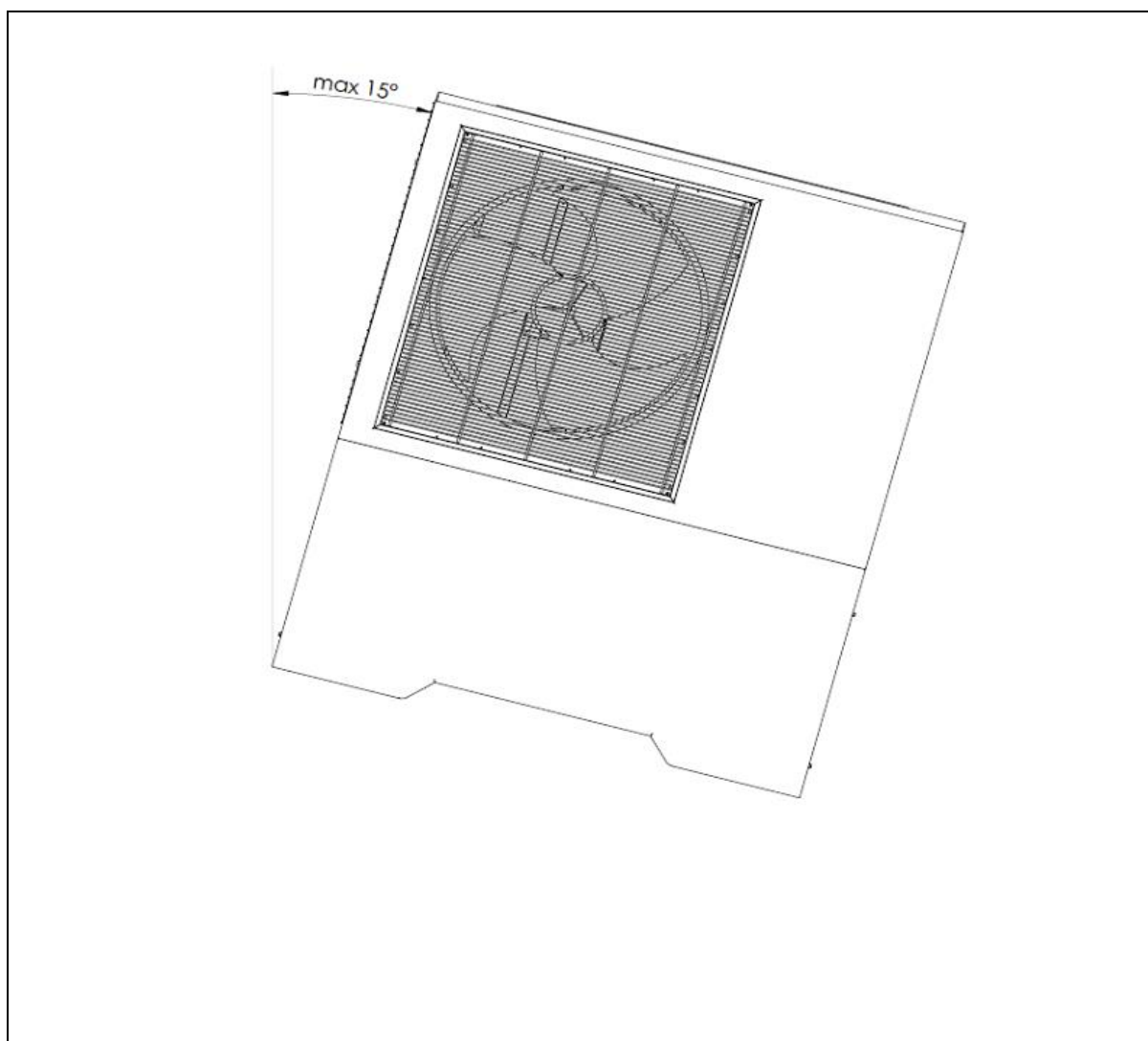
Rys. 7: Maksymalny przechył pompy ciepła EUROS ATMO w czasie transportu.
