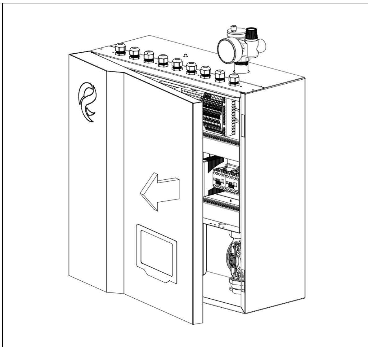
Rys. 13: Sposób otwierania frontowej osłony jednostki wewnętrznej pompy ciepła EUROS ATMO.
