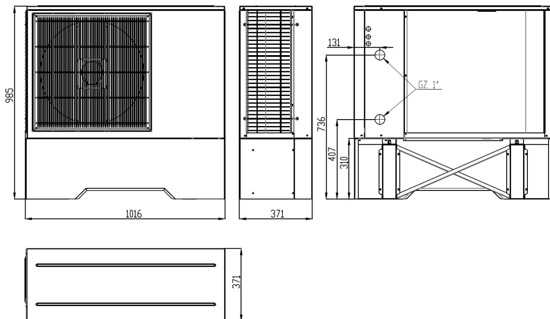
Rys. 8: Gabaryty jednostki zewnętrznej pompy ciepła EUROS ATMO 7
