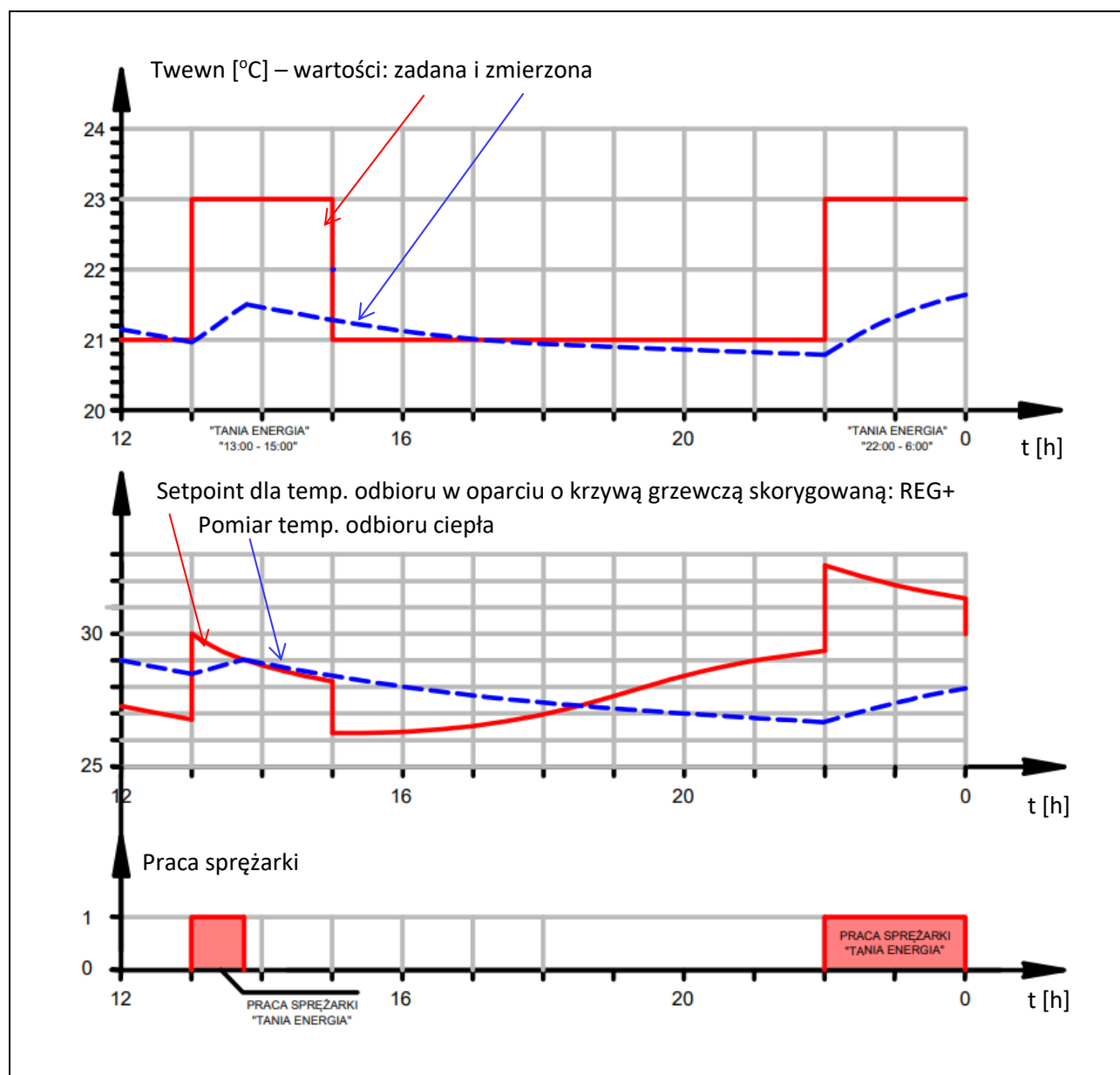
Rys. 27: Automatyczna zmiana temperatury zadanej w trybie ECO z wykorzystaniem mechanizmu REG+.
