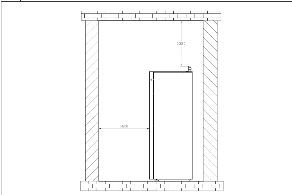
Rys. 13: Ograniczenia dotyczące miejsca ustawienia jednostki wewnętrznej pompy ciepła EUROS HYDRO 200 AIO (wymiary w mm).
