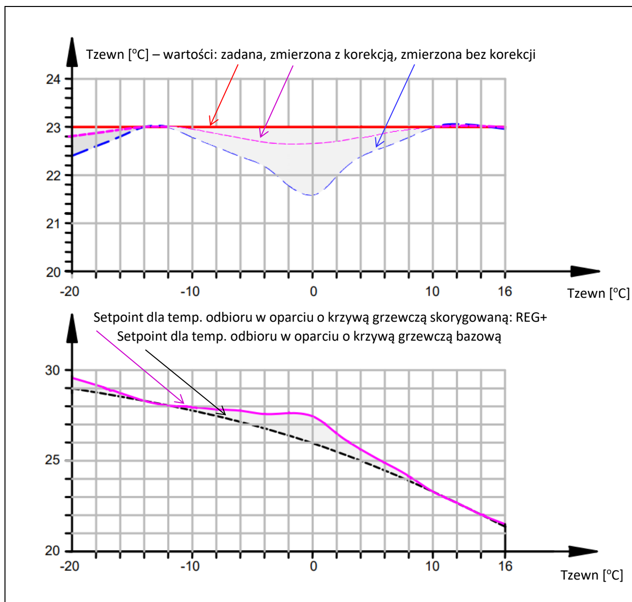
Rys. 25: Oddziaływanie mechanizmu REG+ na krzywą grzewczą.
