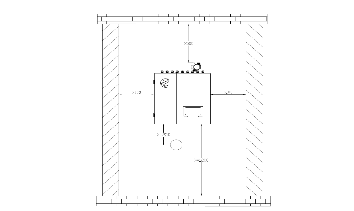
Rys. 12: Ograniczenia dotyczące miejsca ustawienia jednostki wewnętrznej pompy ciepła EUROS ATMO (wymiary w mm).
