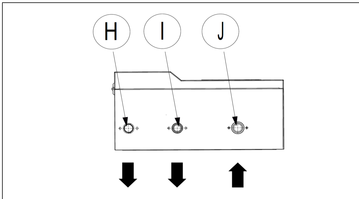
Rys. 16: Przyłącza hydrauliczne jednostki wewnętrznej pompy ciepła EUROS HYDRO 200 AIO.
