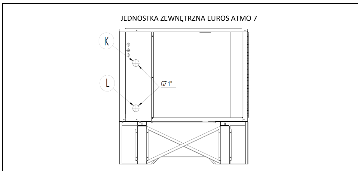
Rys. 17: Przyłącza hydrauliczne jednostki zewnętrznej pompy ciepła EUROS ATMO 7.
