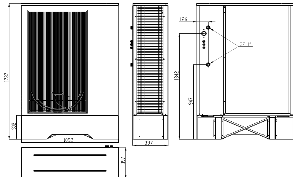
Rys. 11: Gabaryty jednostki zewnętrznej pompy ciepła EUROS ATMO 19
