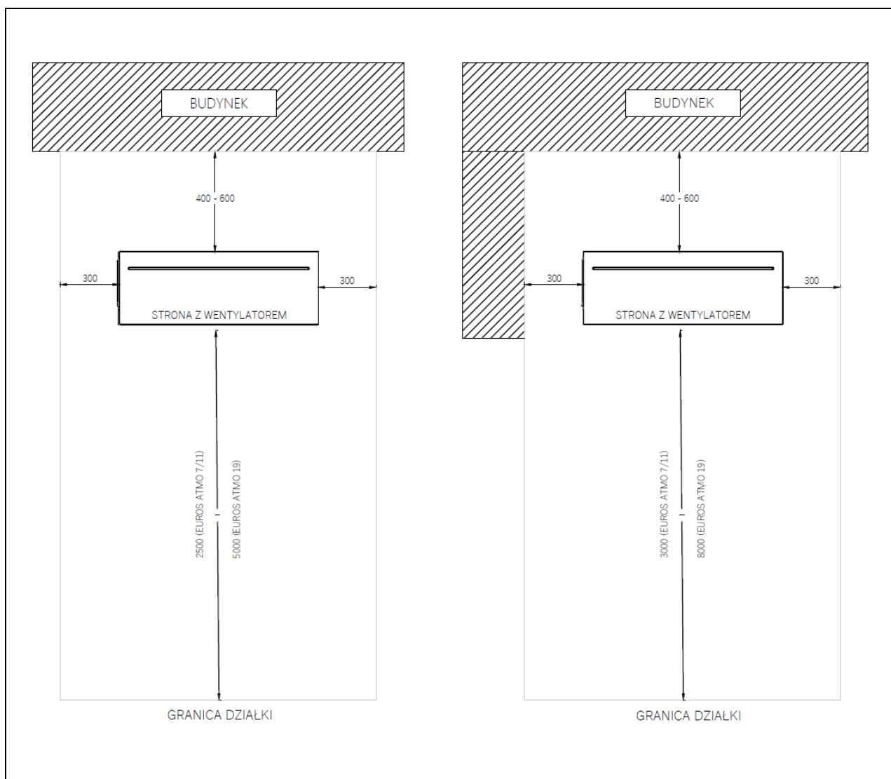
Rys. 14: Ograniczenia dotyczące miejsca ustawienia jednostki zewnętrznej pompy ciepła EUROS ATMO (wymiar w mm).
