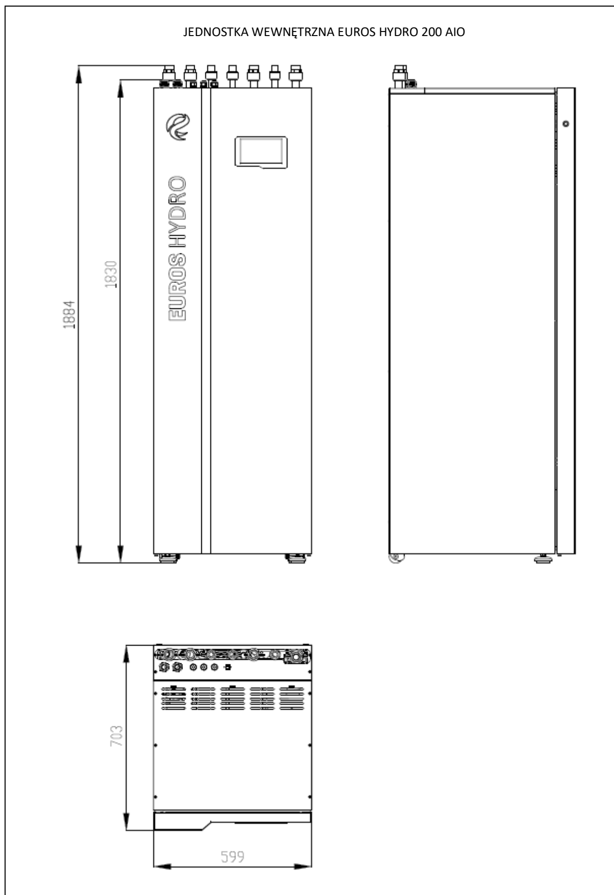
Rys. 7: Gabaryty jednostki wewnętrznej pompy ciepła EUROS HYDRO 200 AIO.
