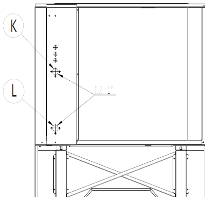
Rys. 18: Przyłącza hydrauliczne jednostki zewnętrznej pompy ciepła EUROS ATMO 11.
